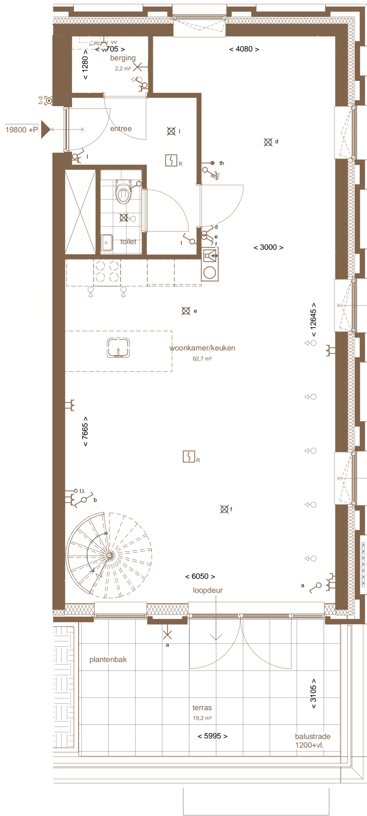
Schaal 1:50
