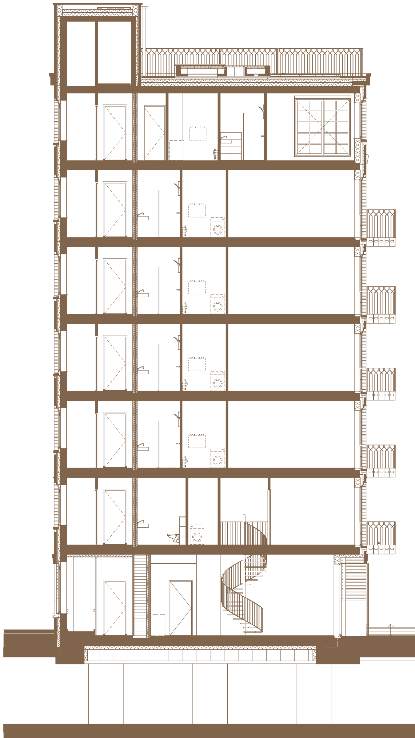
Doorsnede The Bright
