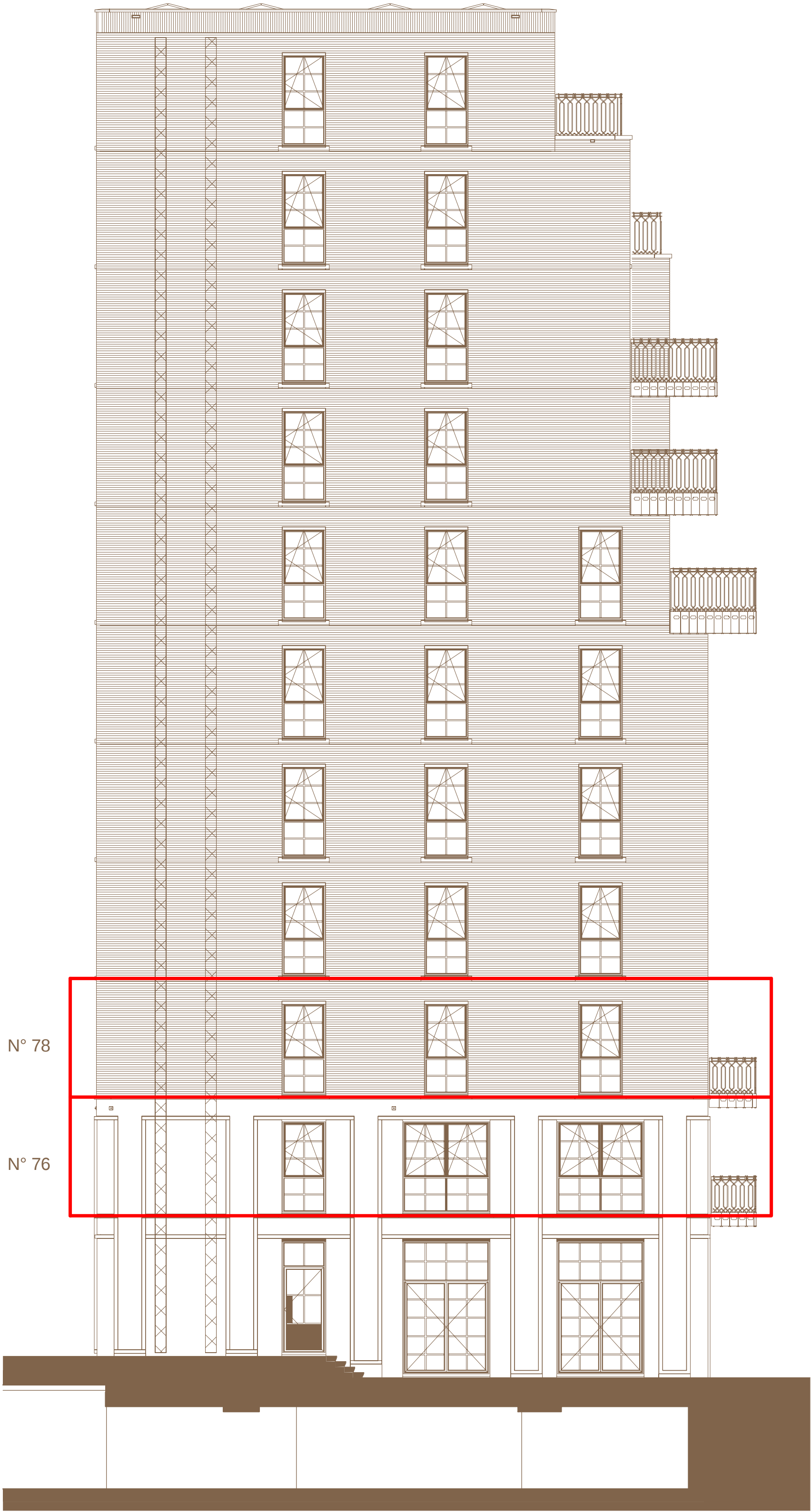
Noordgevel The Regal
